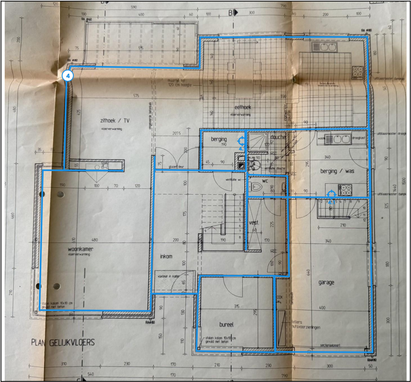
Legende van plan 1.3: Gelijkvloers - muren
