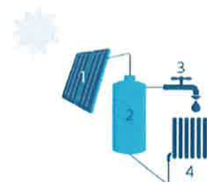
1 Zonnecollector | 2 Opslagvat zonneboiler | 3 Sanitair warm water | 4 Afgegeven warmte voor ruimteverwarming (radiatoren)
