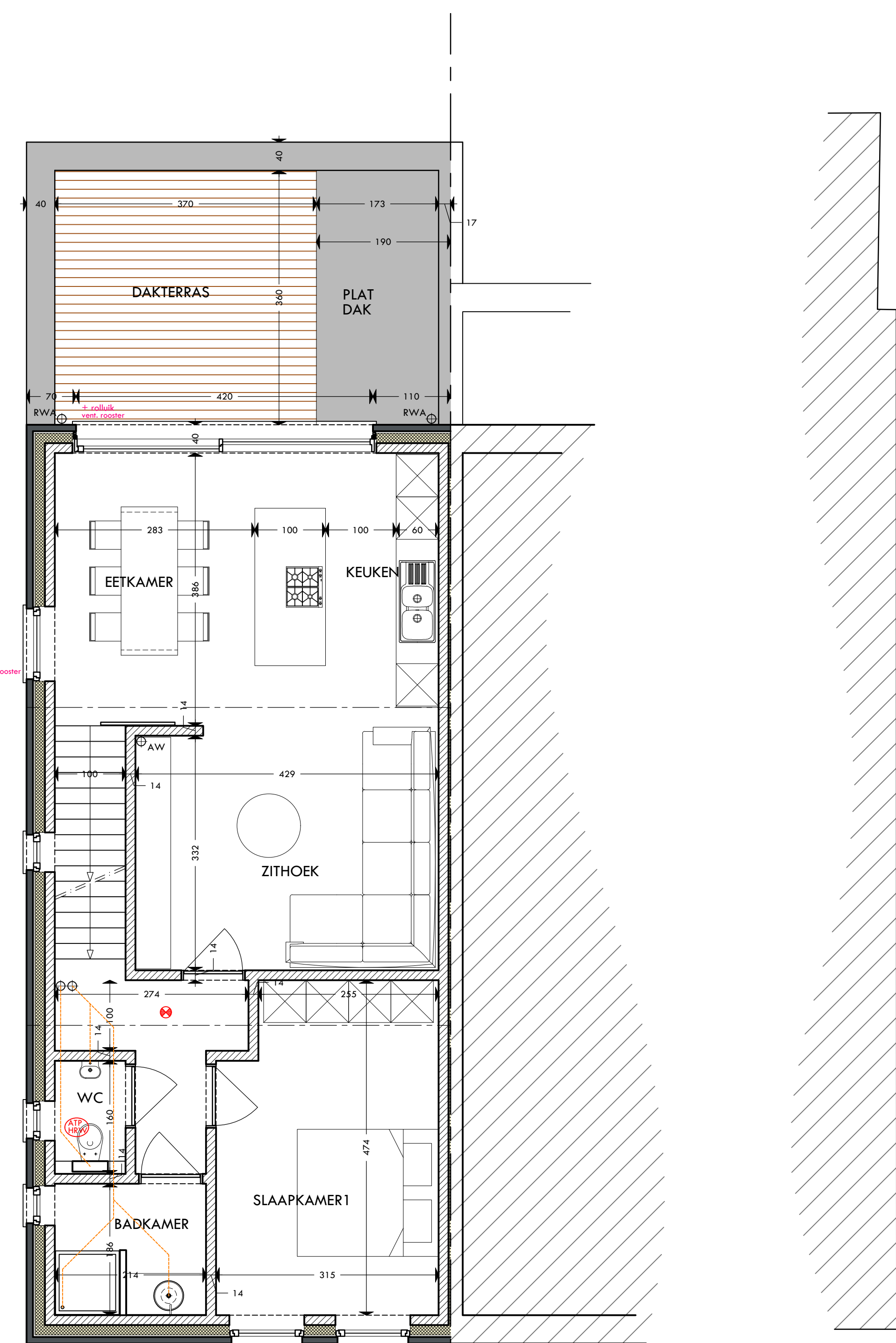
GRONDPLAN VERDIEPING
