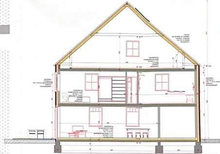
Zijgevel rechts
