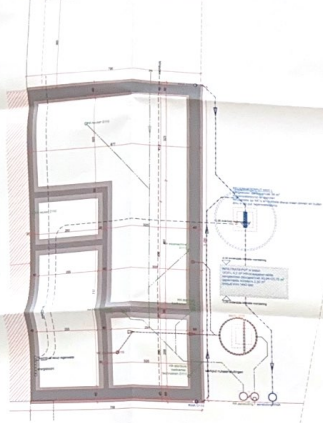
FUNDERINGS- EN RIOLERINGSPLAN
