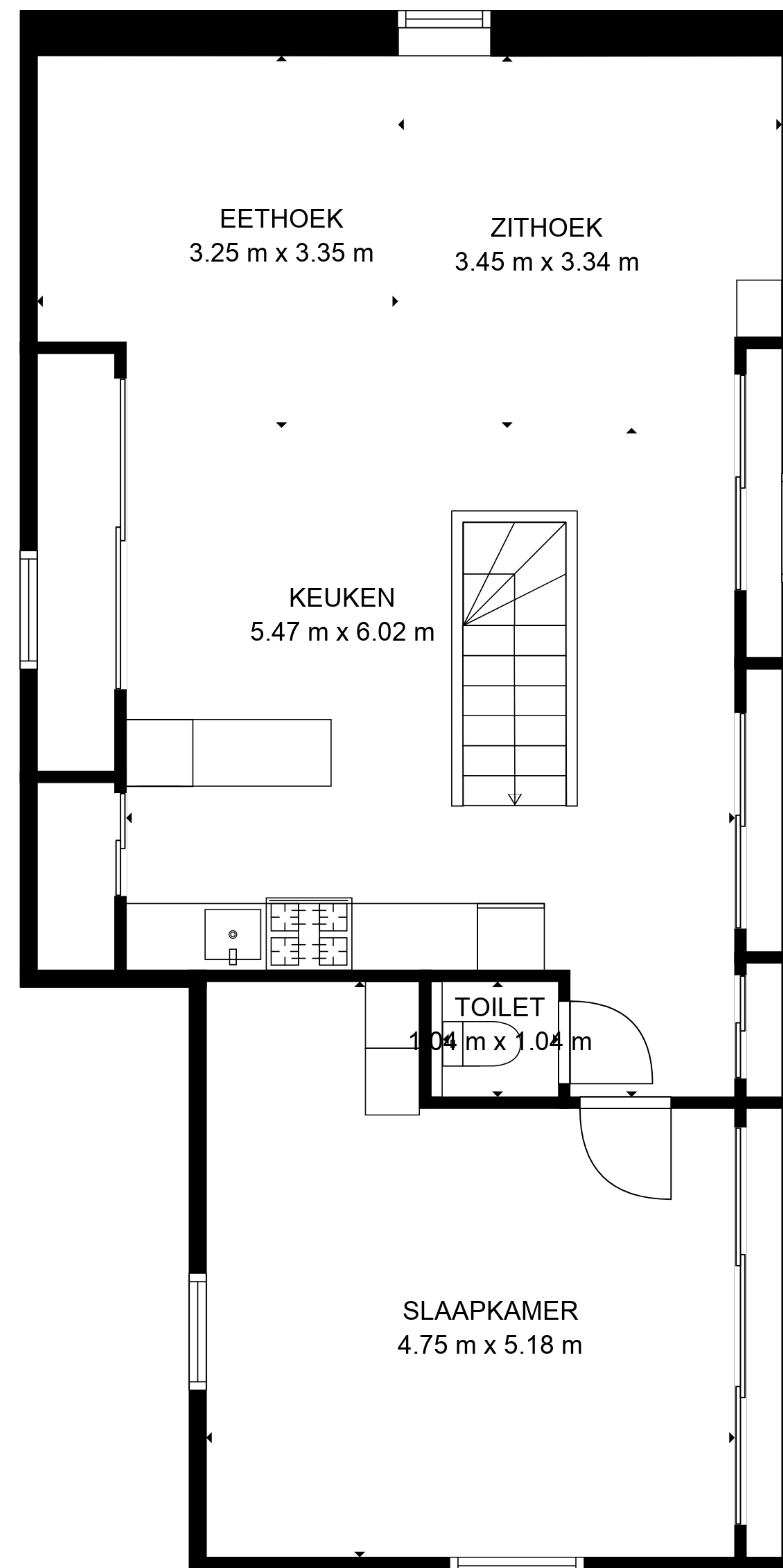
3. VERDIEPING
