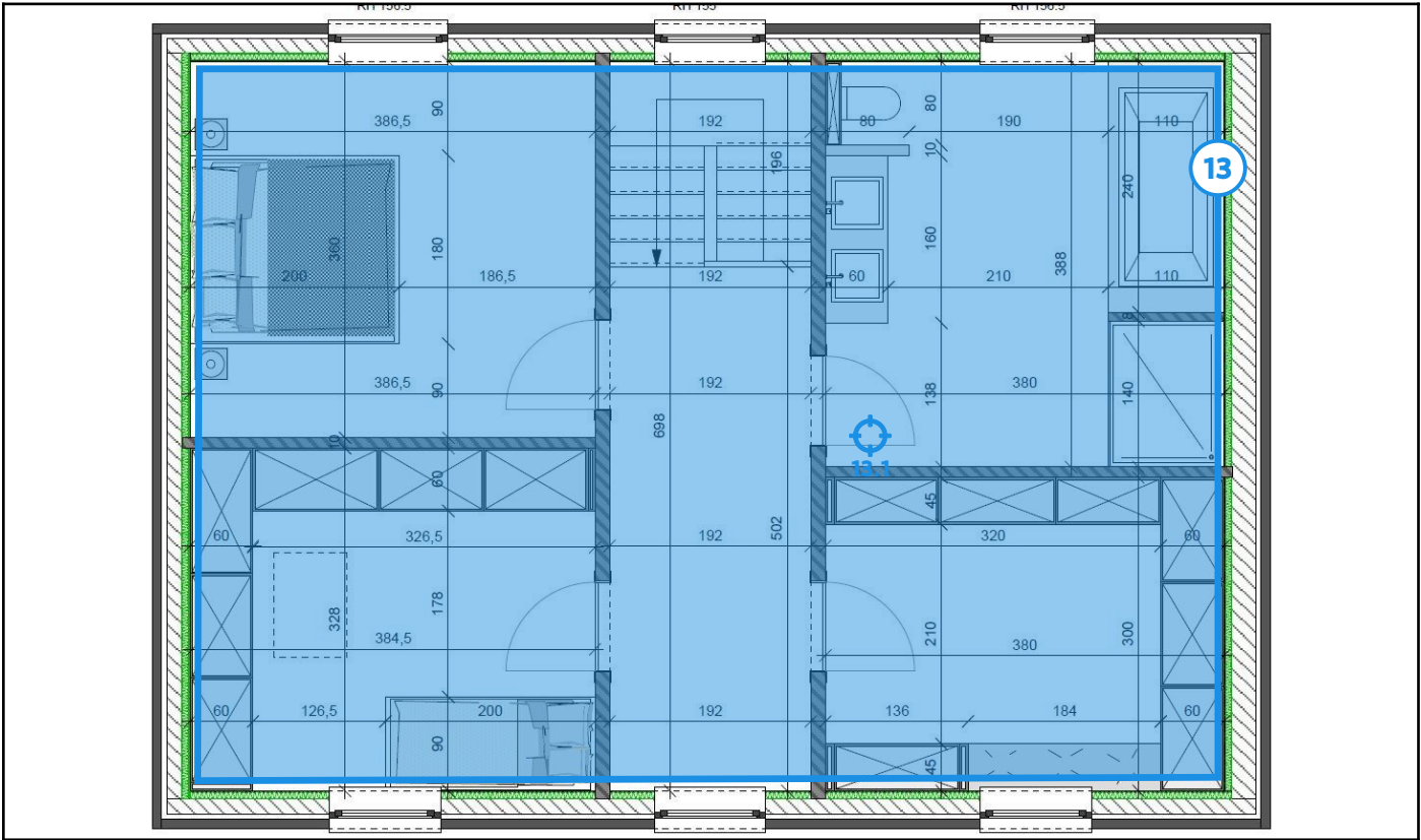
Legende van plan 1.10: Verdieping woonhuis
