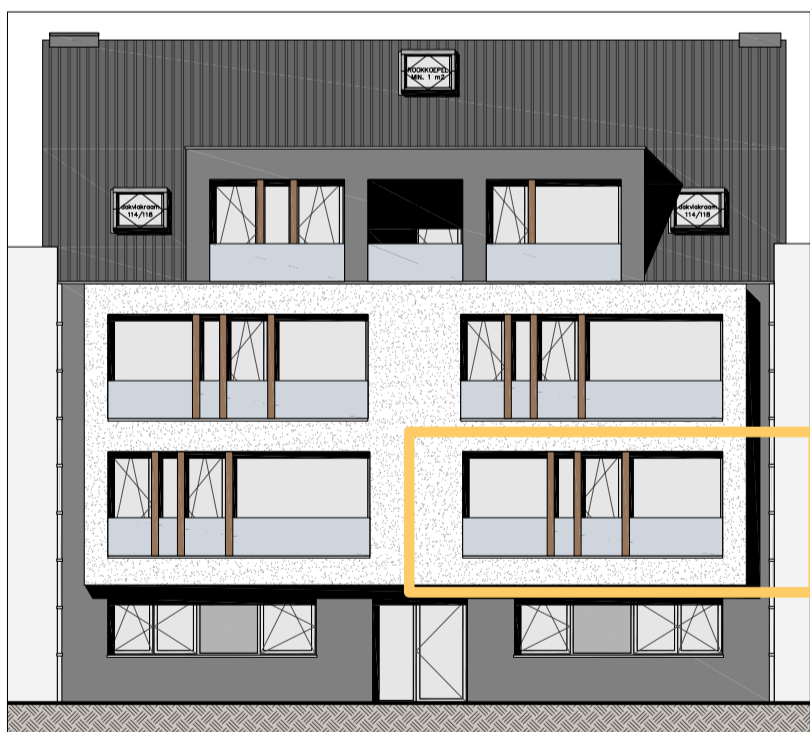
VOORGEVEL
