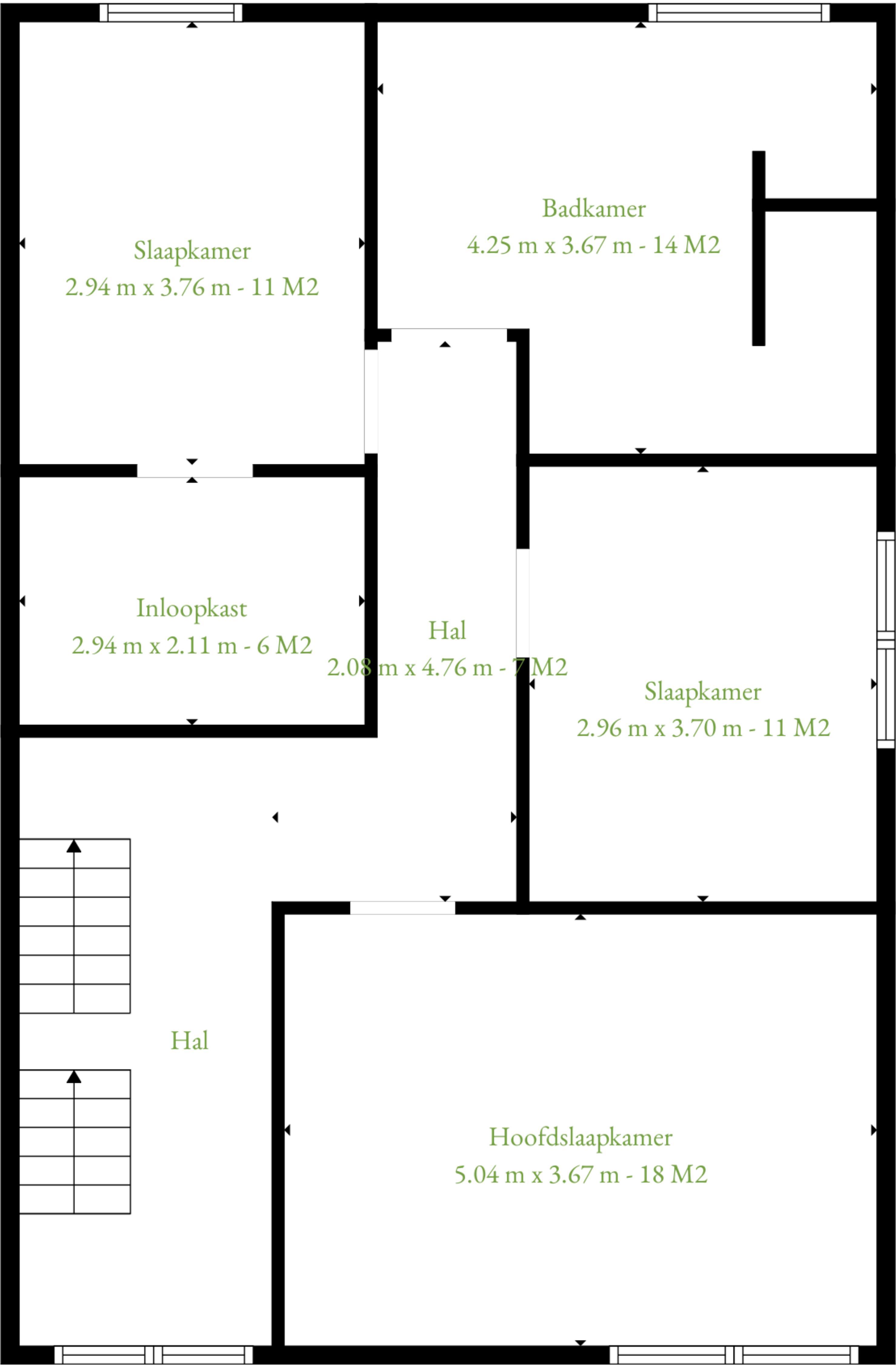
2. Verdieping
