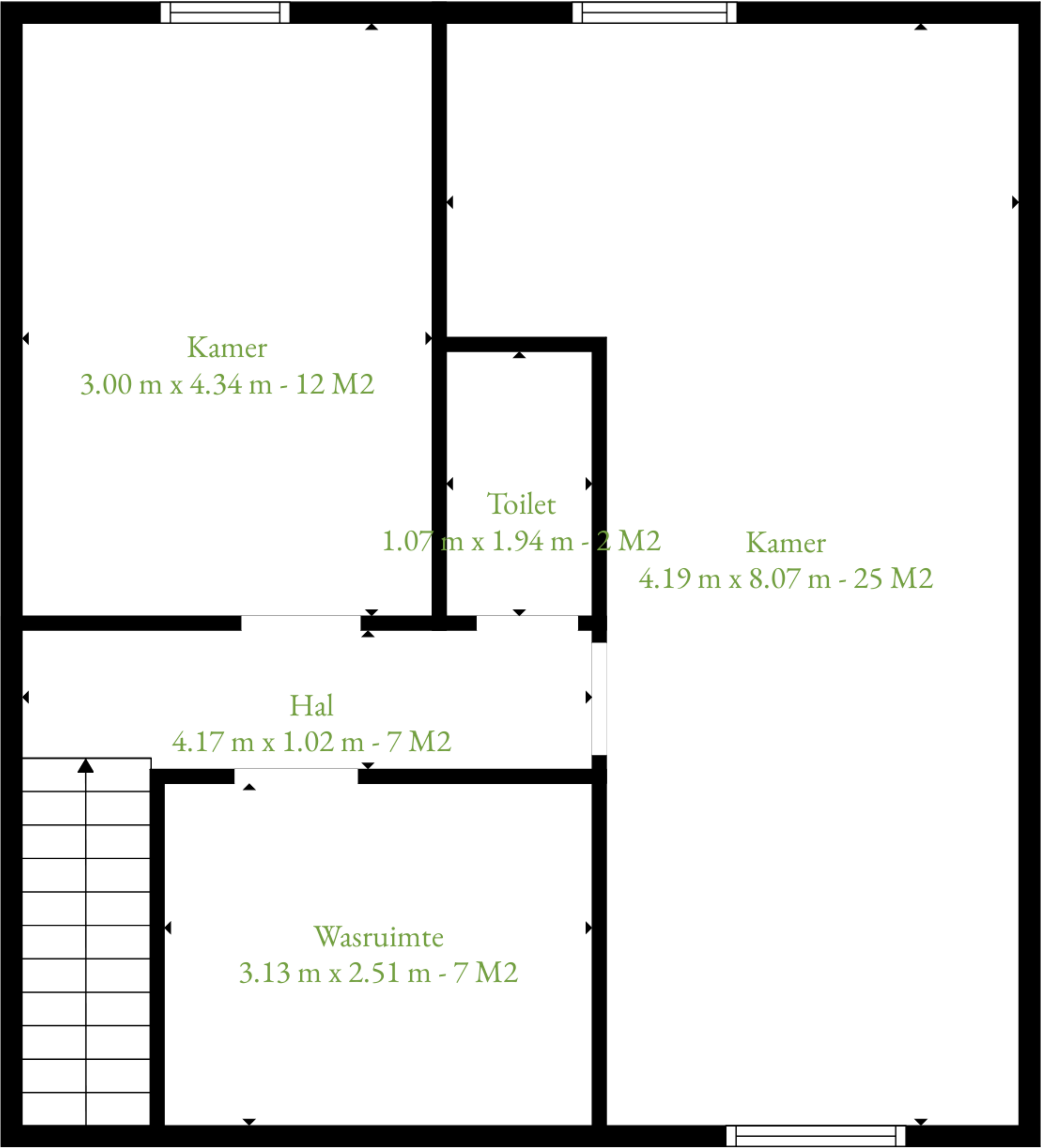
3. Verdieping
